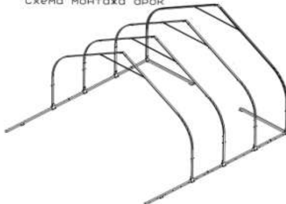
Схема монтажа арок
